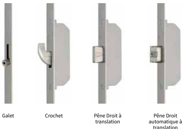
Points de verrouillage additionnels
