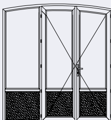
Porte-fenêtre cintré surbaissé
